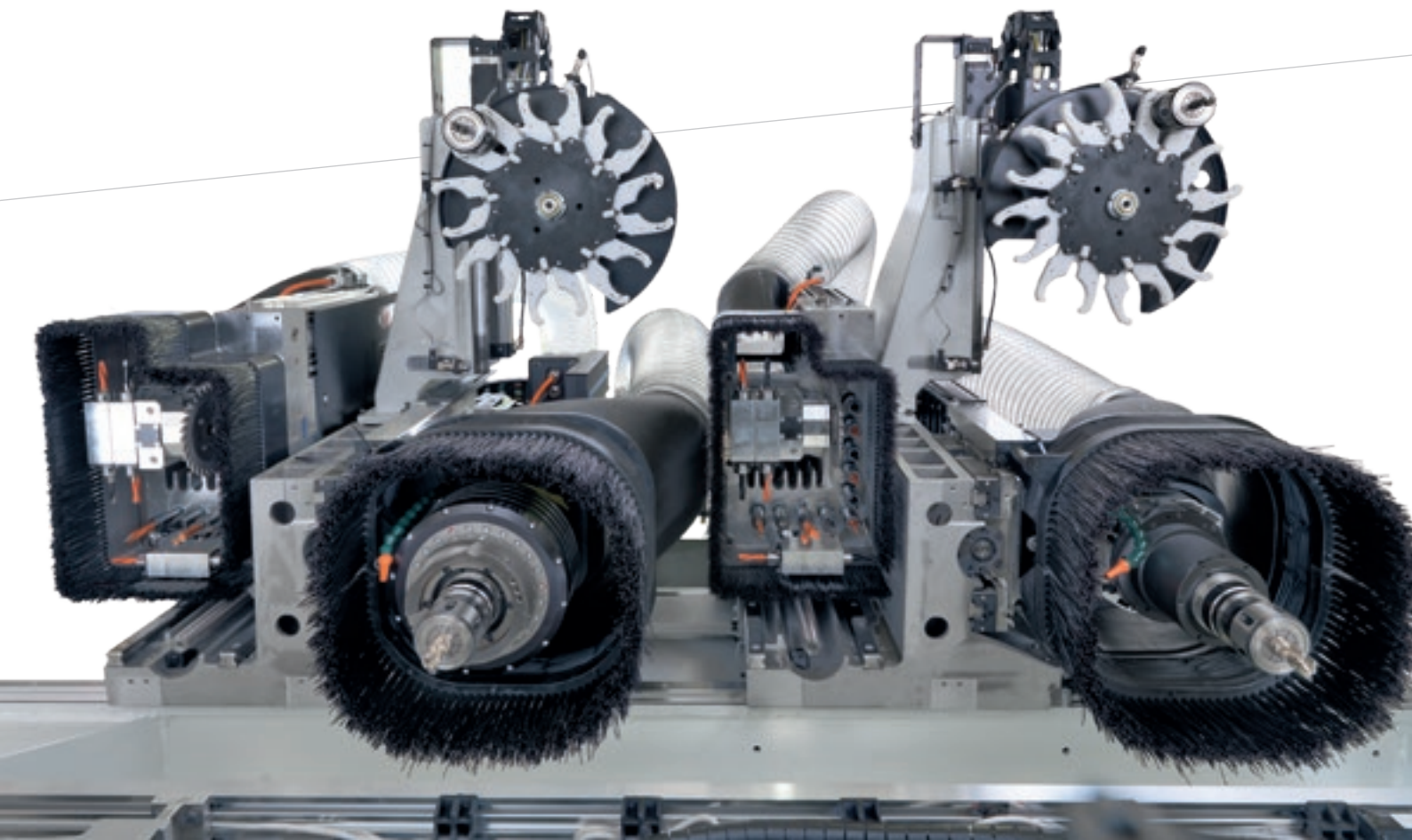
Una configuración para una alta productividad. Mecanizado simultáneo de dos piezas en fresado y taladrado y cambio de herramienta mientras la máquina realiza otras operaciones.
