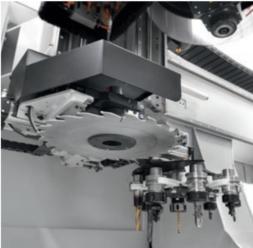
Almacén frontal de puesto individual y almacén herramientas de revolver 8 posiciones
