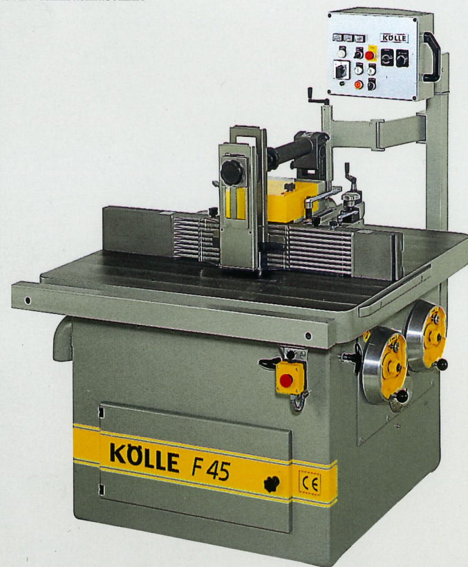
F 45 Schwenkfräsmaschine
