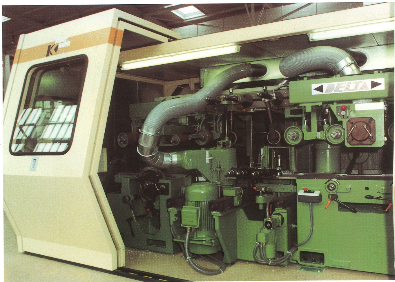
Arbeitseinheit zum horizontalen Spalten bis 300 mm Breite
