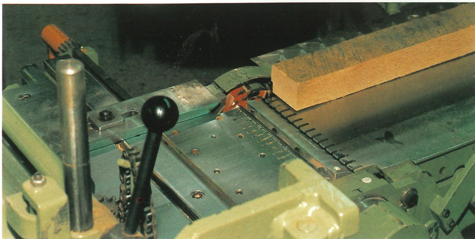
Messerkopf begradigt die untere Fläche, der Fügefräser fräst den Führungsfalz in das Holz.
