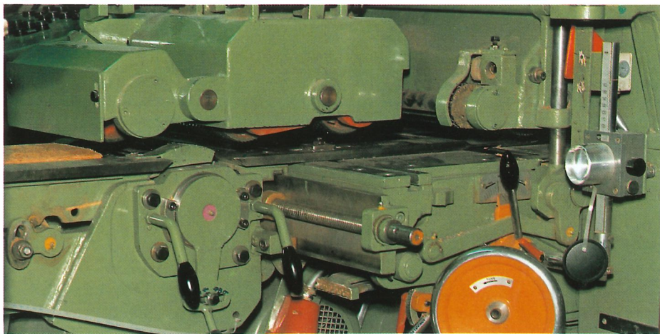
Vorfügende Vorabrichteinheit am Einlauf, um schwierige Arbeitsstücke in einem Durchgang abzurichten und fertig zu bearbeiten.
