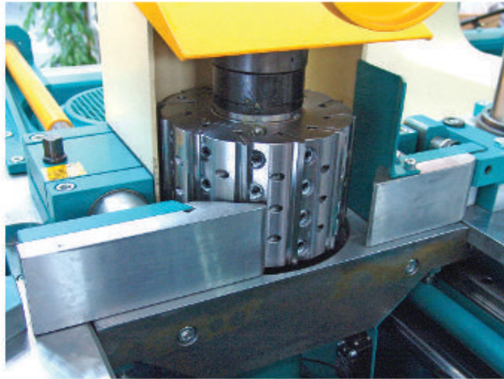
Vertikale Spindeln können auch für Profilarbeiten angepasst werden.
