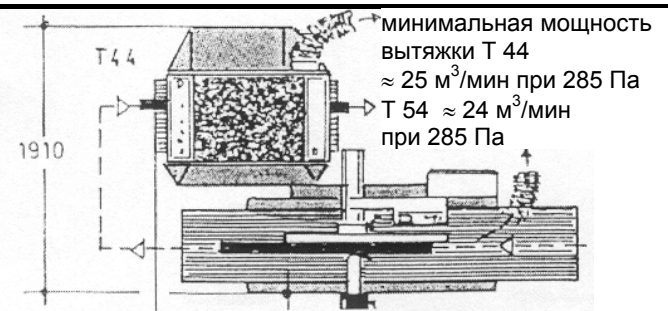
Рейсмусовый станок T 44 и фуговальный станок T 54 в компактном исполнении
