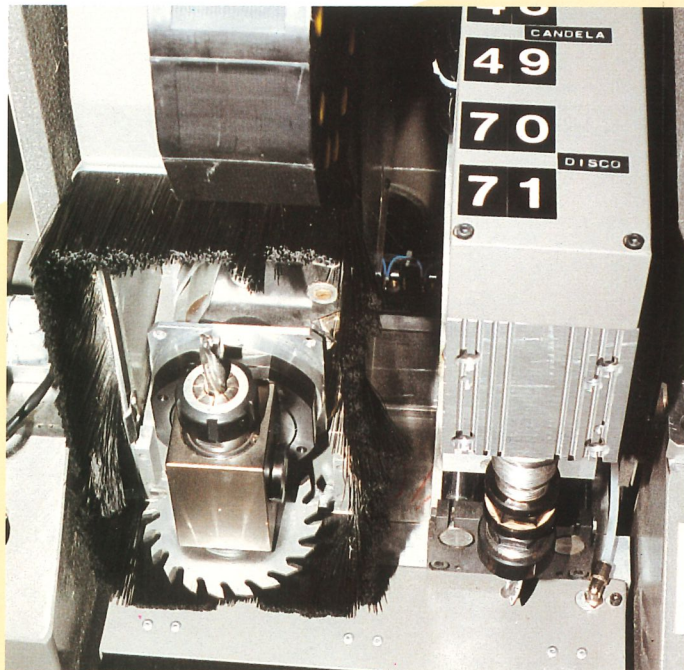
▲ 10 HP Elektro-spindel und Horizontalfräser.
