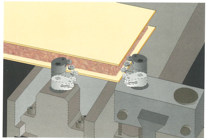
▲ Spezialanschlüge für überfurnierte Werkstücke
