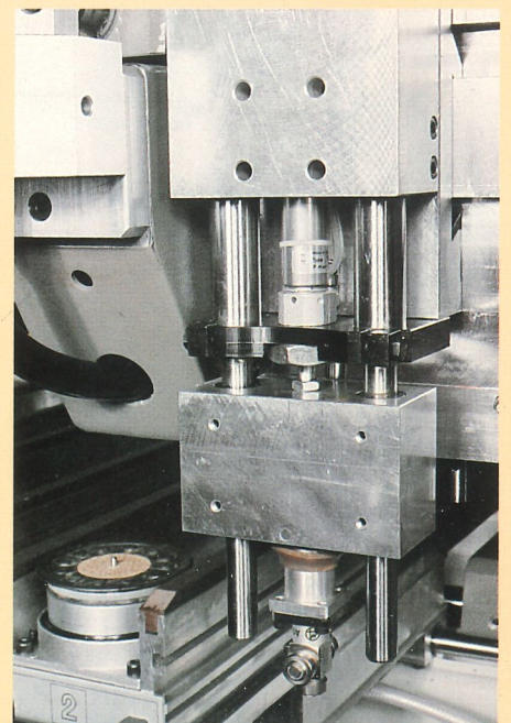
▲ Schwimmend gelagerter Kopf, um der Werkstückoberfläche genau folgen zu können.
