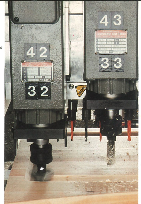
▲ Vertikalfräseinheit mit MK2-Anschluß.
