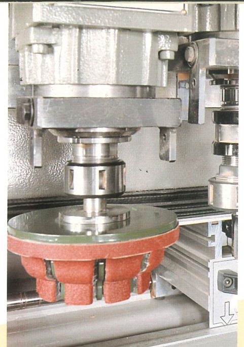
▲ Schleifaggregat.
