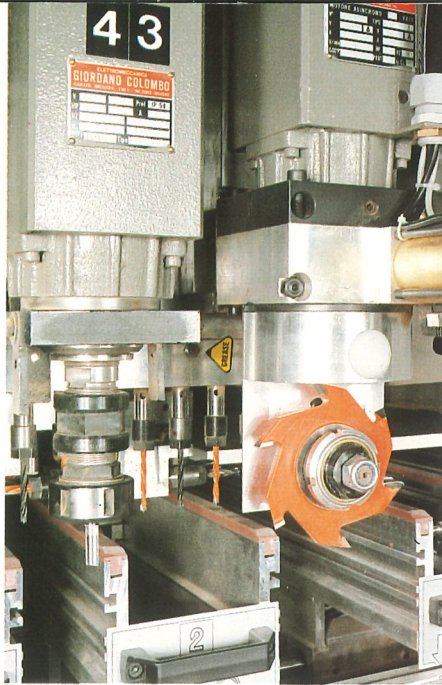
▲ Nutenfräser mit automatischer Drehung.
