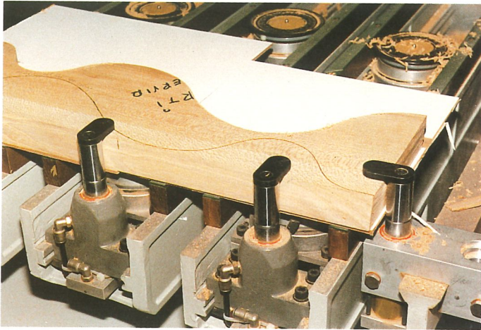
▲ Blockierung des Werkstückes durch Niederhalter
