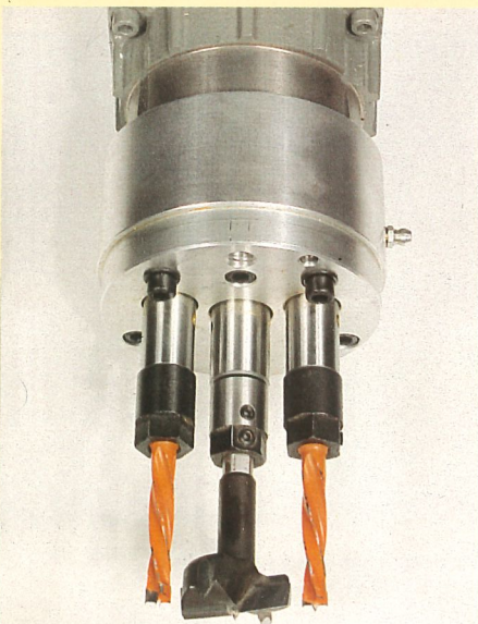
◀ Bohreinheit für Scharniere.
