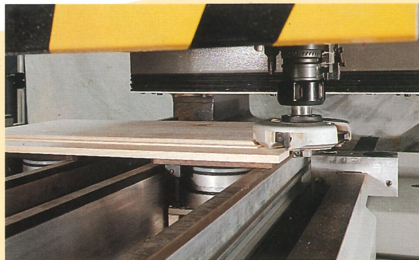
▼ Bearbeiten eines Fensterflügels
