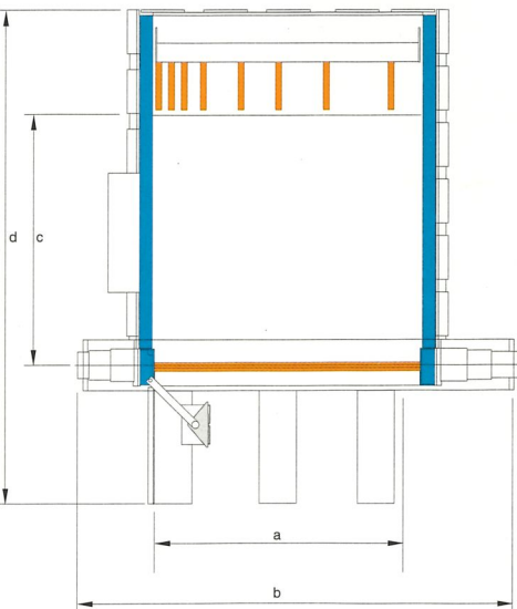
Maße/Dimensions - mm
