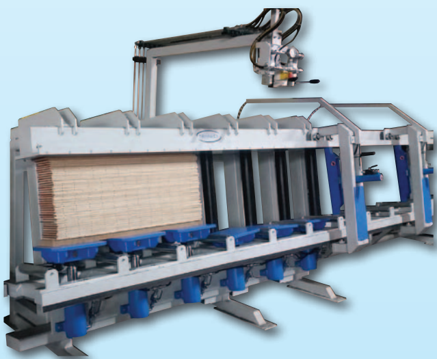
Side rotor for parquet lamelas Seitigenrotor für den Parkettlamellen Rotor latéral pour l'assemblage des lames de parquet Rotore laterale per l'incollaggio delle lamelle del parquet Rotor lateral para pegar las lamelas de parqué Боковой ротор для склеивания паркетных ламелей
