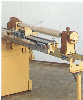
Drehstuhl-Einrichtung
