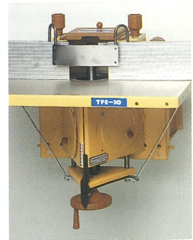
Tischfräs-Einrichtung
