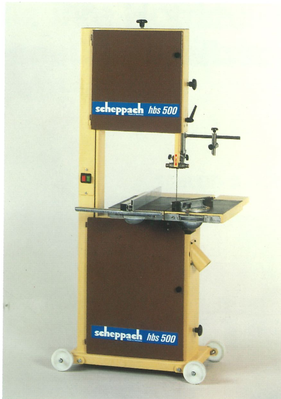
hbs 500 mit Sonderzubehör
