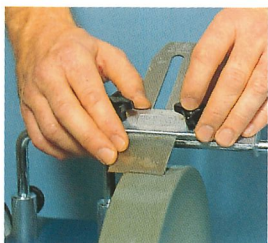
Schleifvorrichtung SVH-60 für Hobeisen
