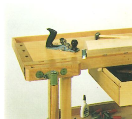
Hobelbank
