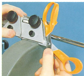
Schleifvorrichtung SVX-150 für Scheren
