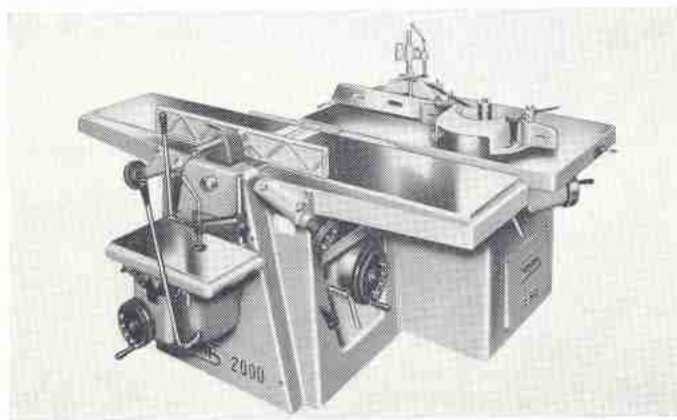
Kombinierte Universalmaschine, auch getrennt verwendbar, Modell 2000
