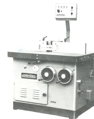
Schwere Schwenfräsmaschine Shaper-Tilttable Spindle Toupie lourde à arbre inclinable
