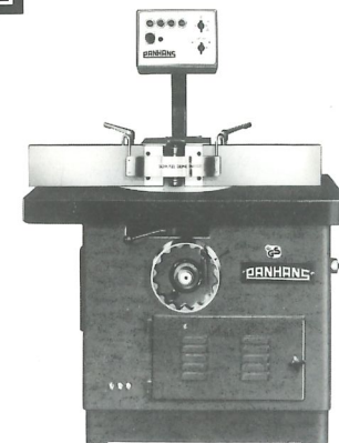
Schwere Starrfräsmaschine Shaper-Fixed Spindle Toupie lourde
