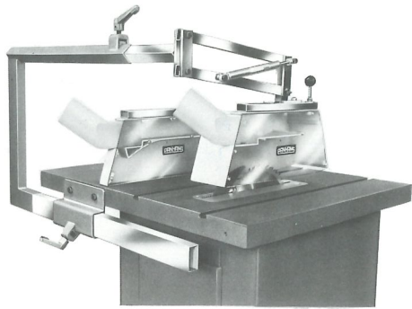
Kreissägen-Schutzvorrichtung Circular saw protective device Dispositif de protection pour scies circulaires
