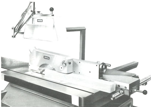
Vorschubapparat Feeding apparatus Appareil d'avance
